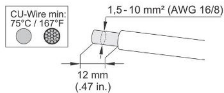
Abbildung 5: Push-in Federzugklemme und Anforderungen an das Kabel zur Installation des PV Points
