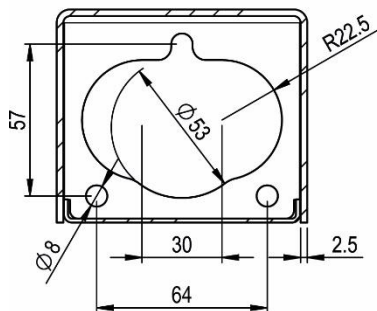
A-A (1 : 2)
